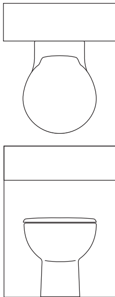
Space 60cm wc unit w600 x h800 x d210mm
