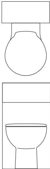
Space 45cm wc unit w450 x h800 x d210mm
